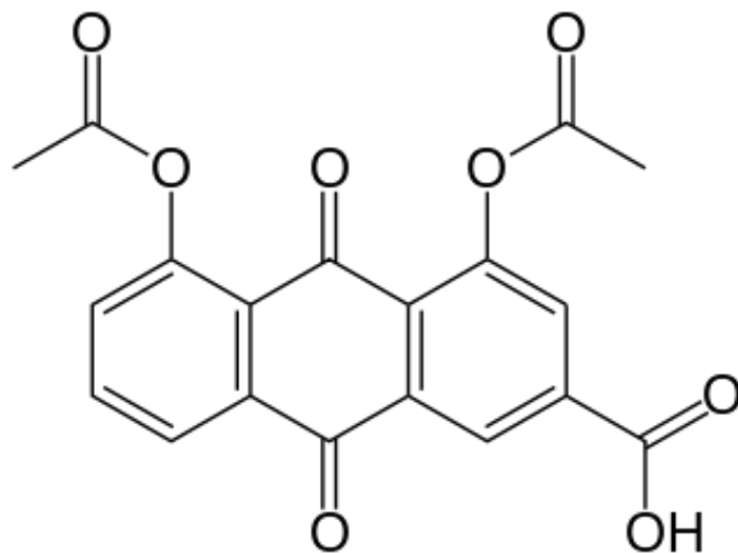
Diacetyl rhein (diacerein)
